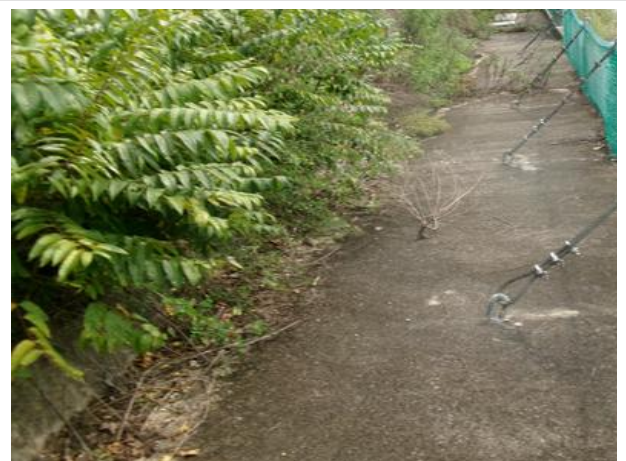
소단배수로 토사퇴적
